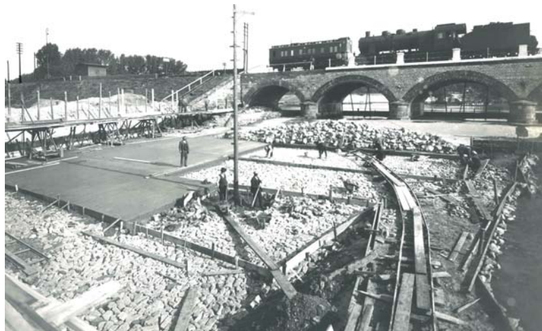
Budowa jazu (zakładanie płyty betonowej) przy ujęciu wody na Białej Przemszy w Maczkach – 1.10.1929 r. Zdjęcie pochodzi ze strony internetowej: www.gpw.katowice.pl
