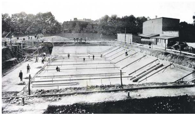
Budowa zbiornika wodociągowego na Mecu (Metzu) w Zagórz. W tle widać dziewiętnastowieczny pałac Malplata (ul. Braci Mieroszewskich 7). Zdjęcie zostało udostępnione przez GPW Katowice.
